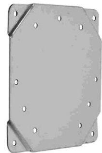
Montage-Platte Typ A-368 Maße: 130 x 130 mm Material: Alu-Blech
