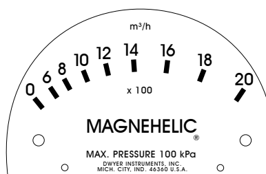
Volumenstrom-Messung
